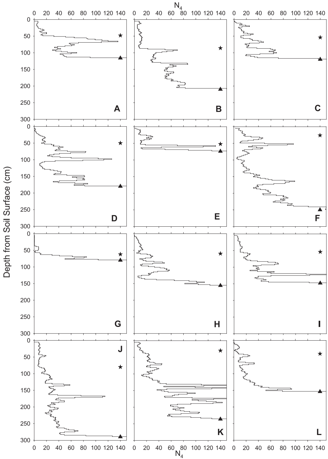
図-5 土壌硬度の鉛直分布 ★ I層の下端, ▲ II層の下端・III層の上端
