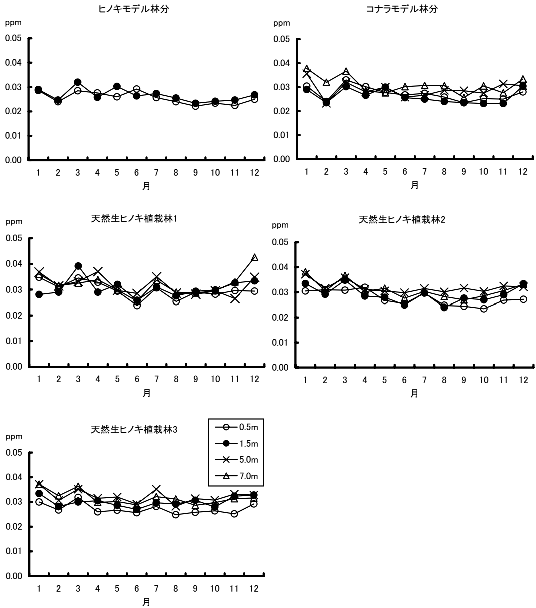
図-9 測定高ごとの月別の平均NO 2 濃度
