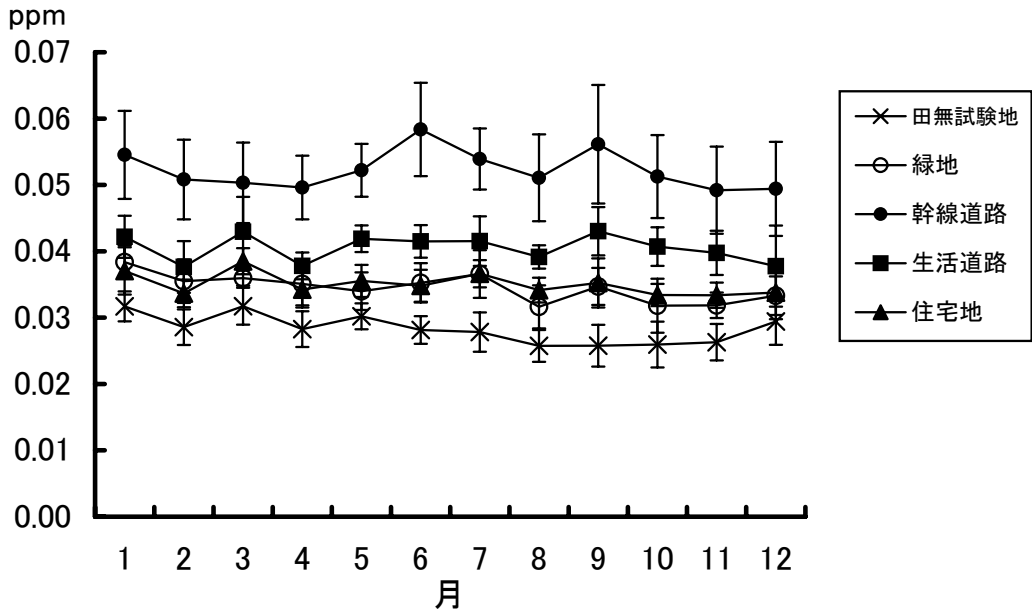
図-5 グループごとの月別平均NO 2 濃度
